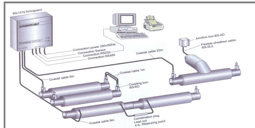
Systemy rozpoznawania i lokalizowania przecieków: BRANDES
